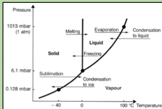
Frysetørringsprocessen
